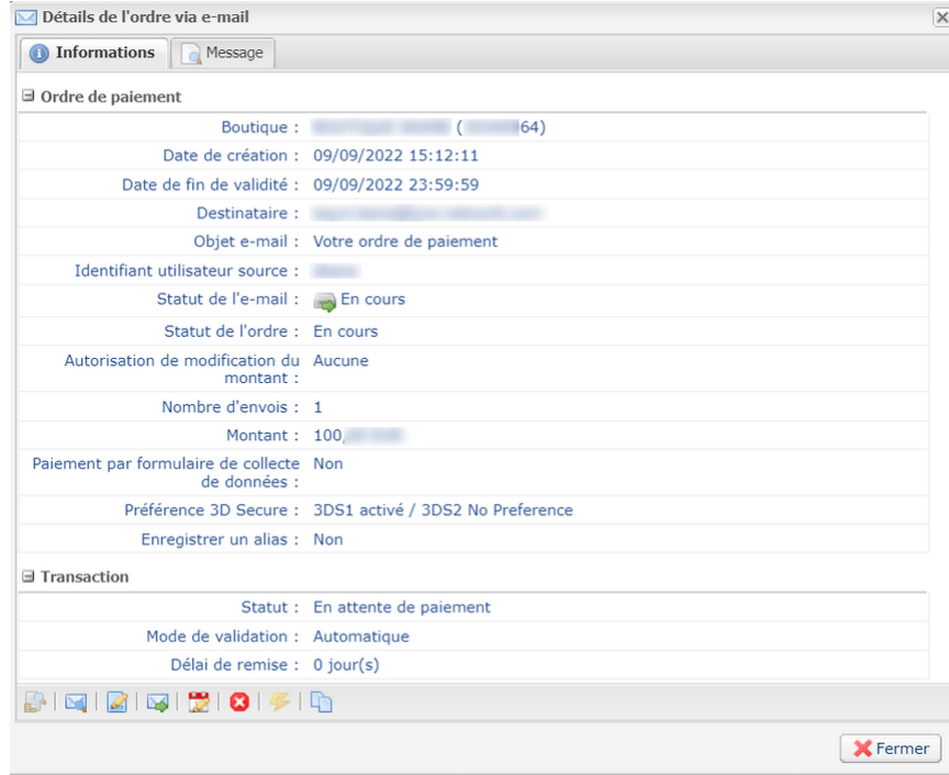
Image 1 : Onglet Informations
